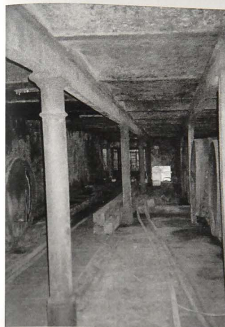
7. kép Az 1909-es évszámmal jelzett szárny acélfödémekkel és oszlopokkal. A padozaton futó sínrendszert ma is használják (Dr. Lukács László felvétele, 2016.)
